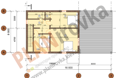
План другого поверху м 1:100
