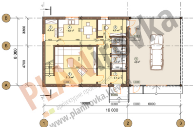
План першого поверху м 1:100
